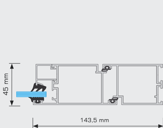
Tür - Querschnitt
