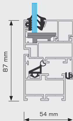
Fenster - Querschnitt
